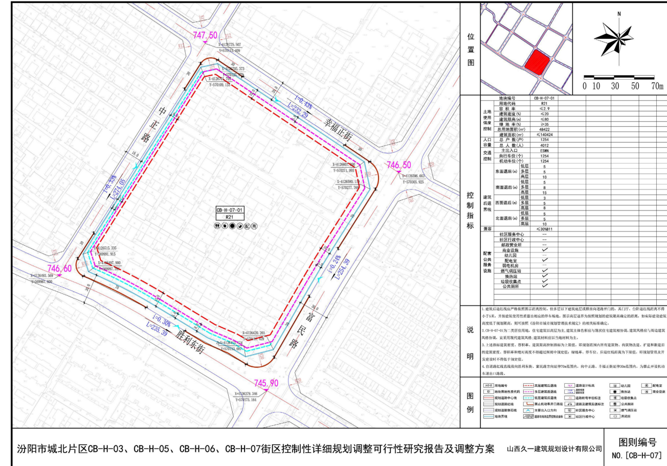
调整后 CB-H-07 图则
