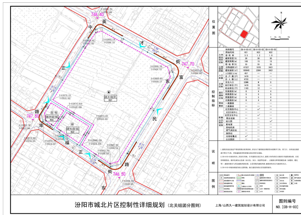
原控规 CB-H-03 图则
