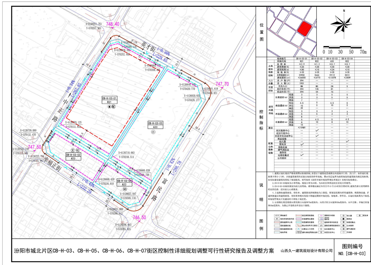
调整后 CB-H-03 图则
