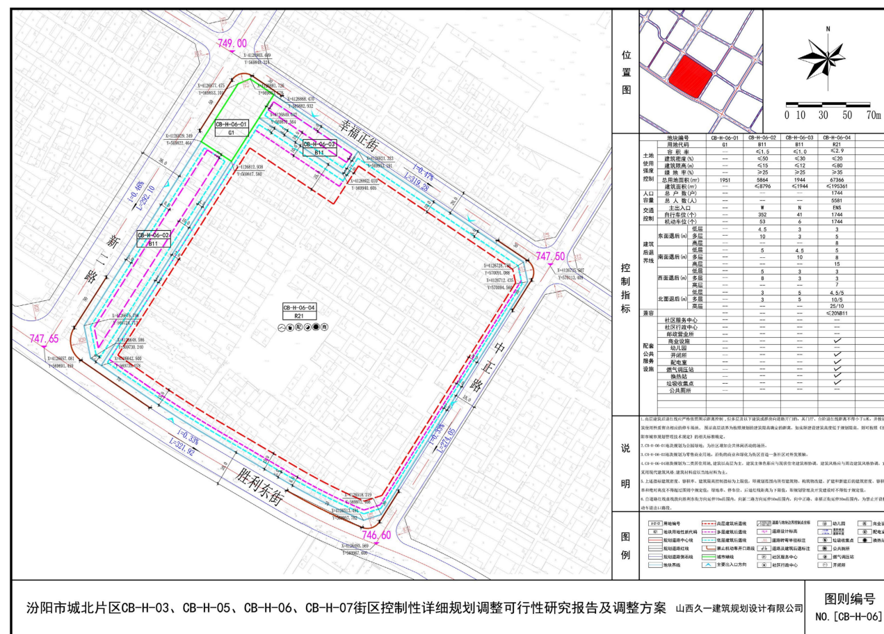
调整后 CB-H-06 图则
